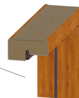
Ościeżnica z blachy aluminiowej z rdzeniem z drewna klejonego wraz z uszczelką.
